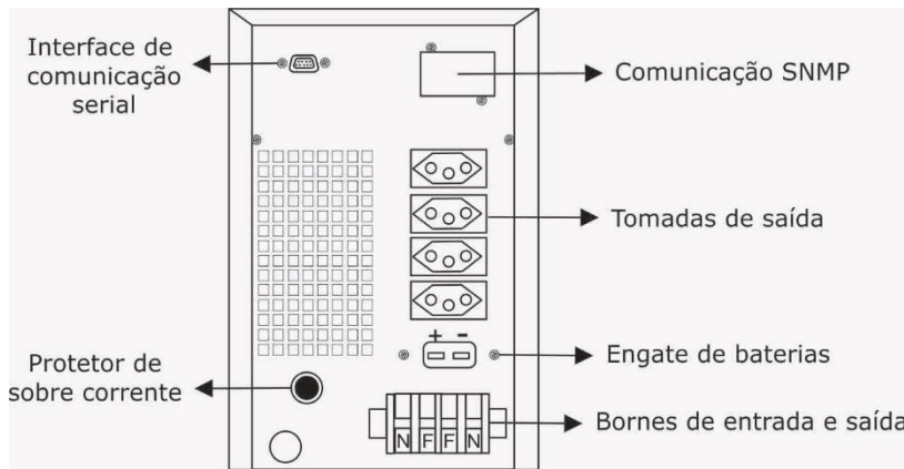
Nobreak 2, 3 e 4kva – MS 2000 | MS 3000 | MS 4000
