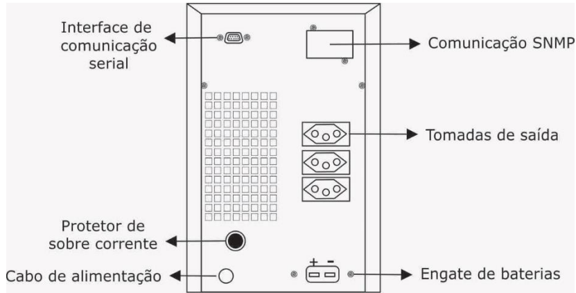
Nobreak 1kva - MS 1000
