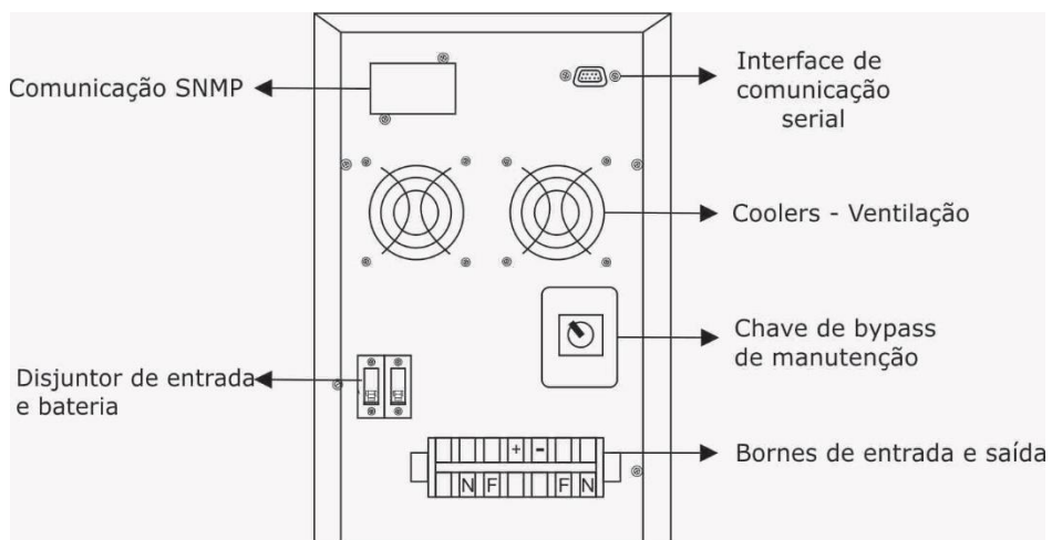
Nobreak 6 – 20kva MS 6000 à MS 20000
